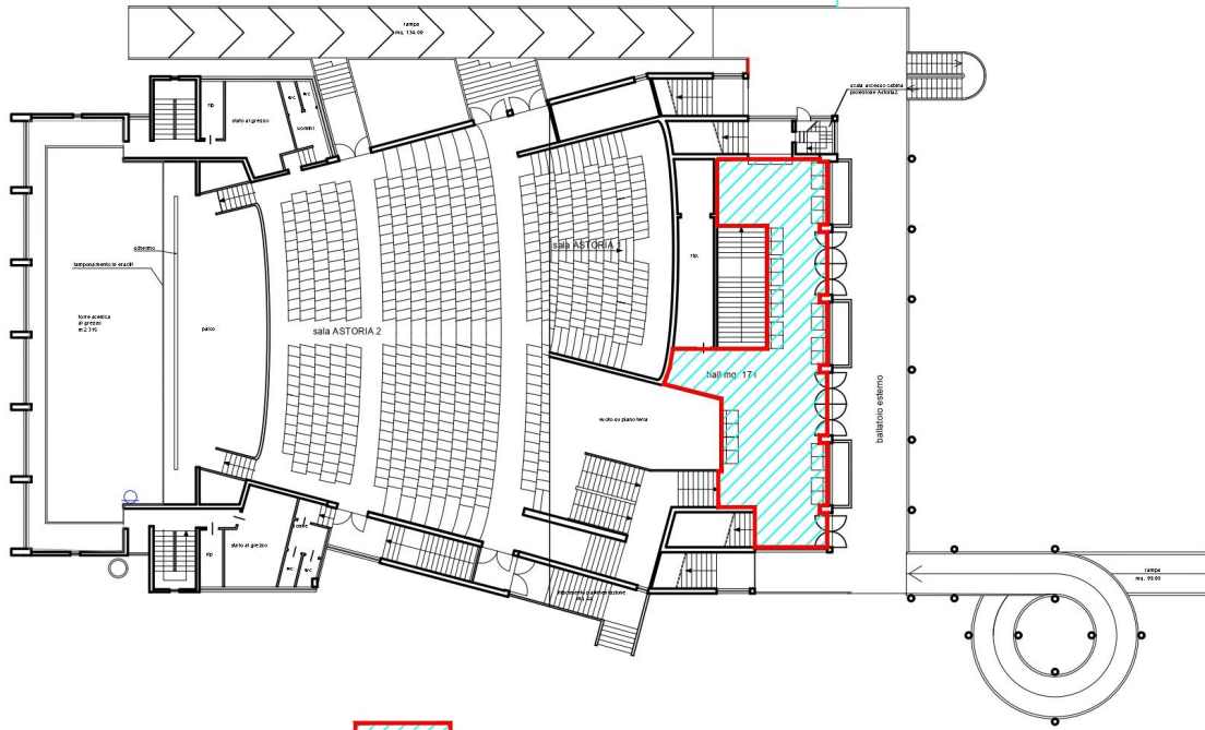
PIANO QUOTA ml. 5,00 - Scala 1:100
