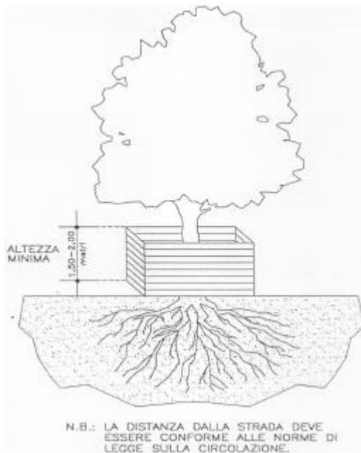
Fig. 11: Protezione dell'albero attraverso la delimitazione dell'area minima di rispetto per alberature stradali con poco spazio.
