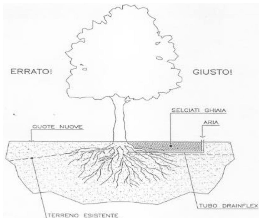
Fig. 4 Accorgimenti per l'innalzamento della quota di terreno nelle aree di pertinenza delle alberature. La ricarica di terreno nelle aree di pertinenza degli alberi è vietata.
