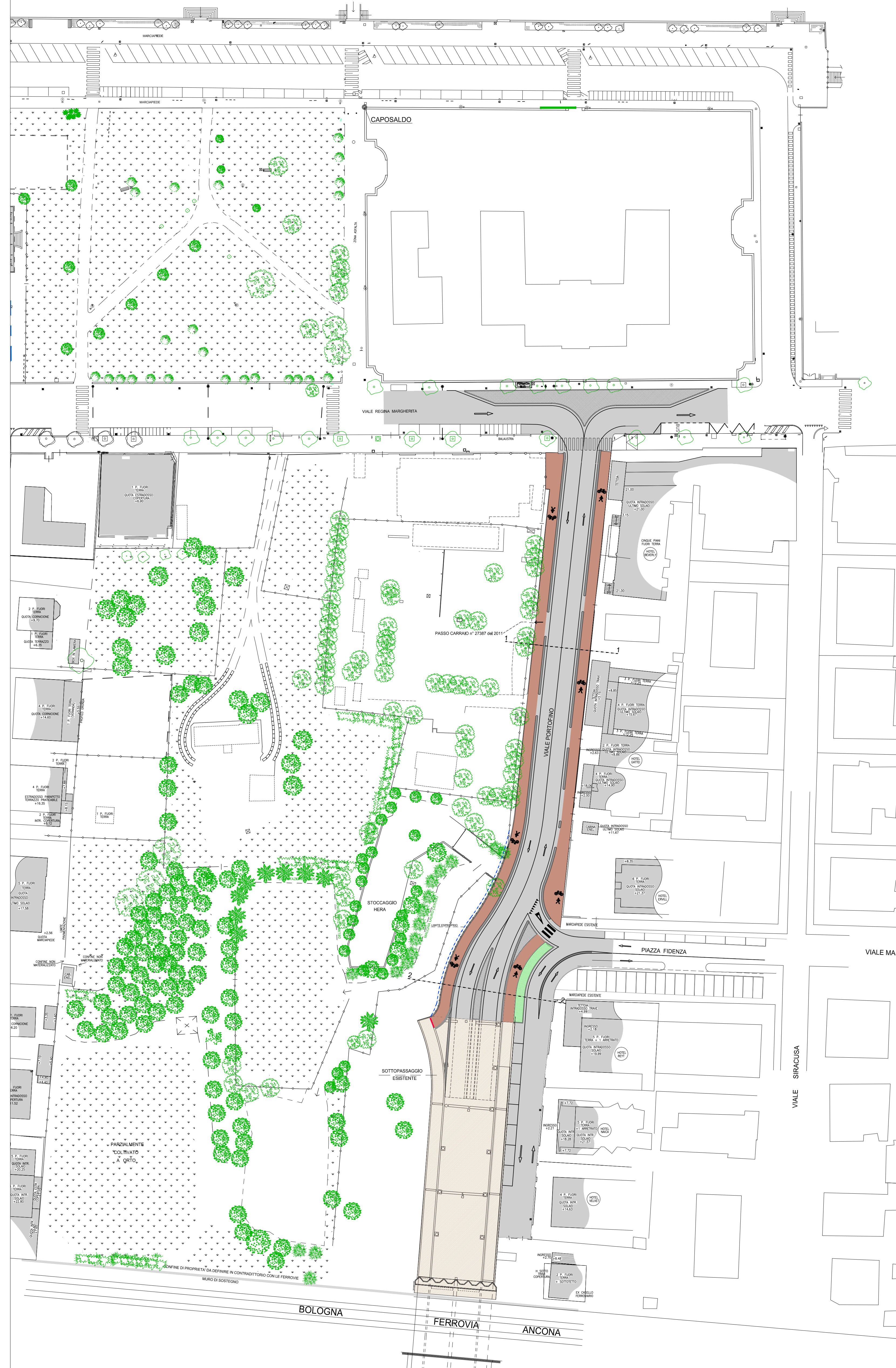
PLANIMETRIA DI PROGETTO scala 1:500
