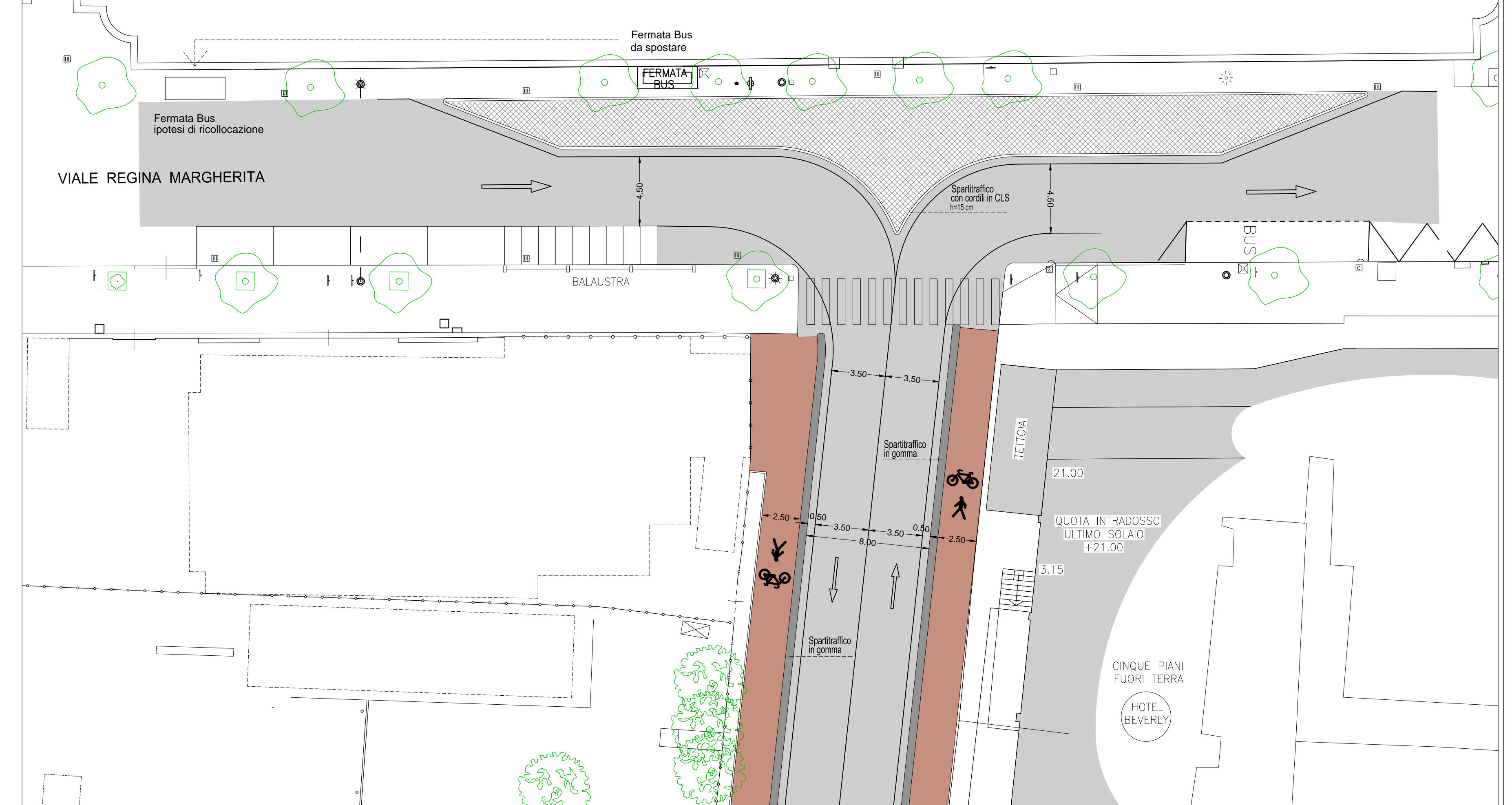
PLANIMETRIA DI PROGETTO particolare 2 scala 1:200
