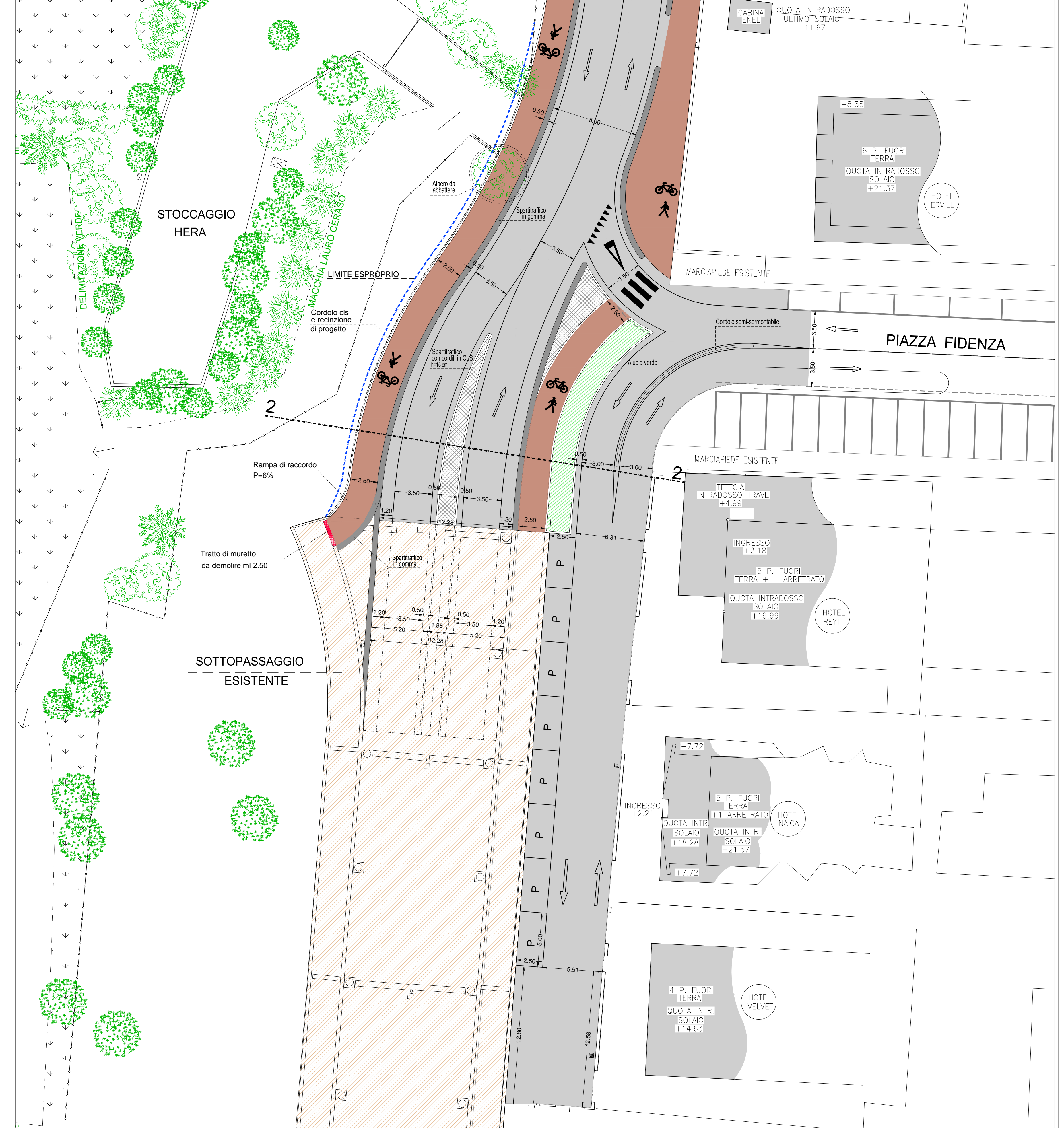
PLANIMETRIA DI PROGETTO particolare 2 scala 1:200
