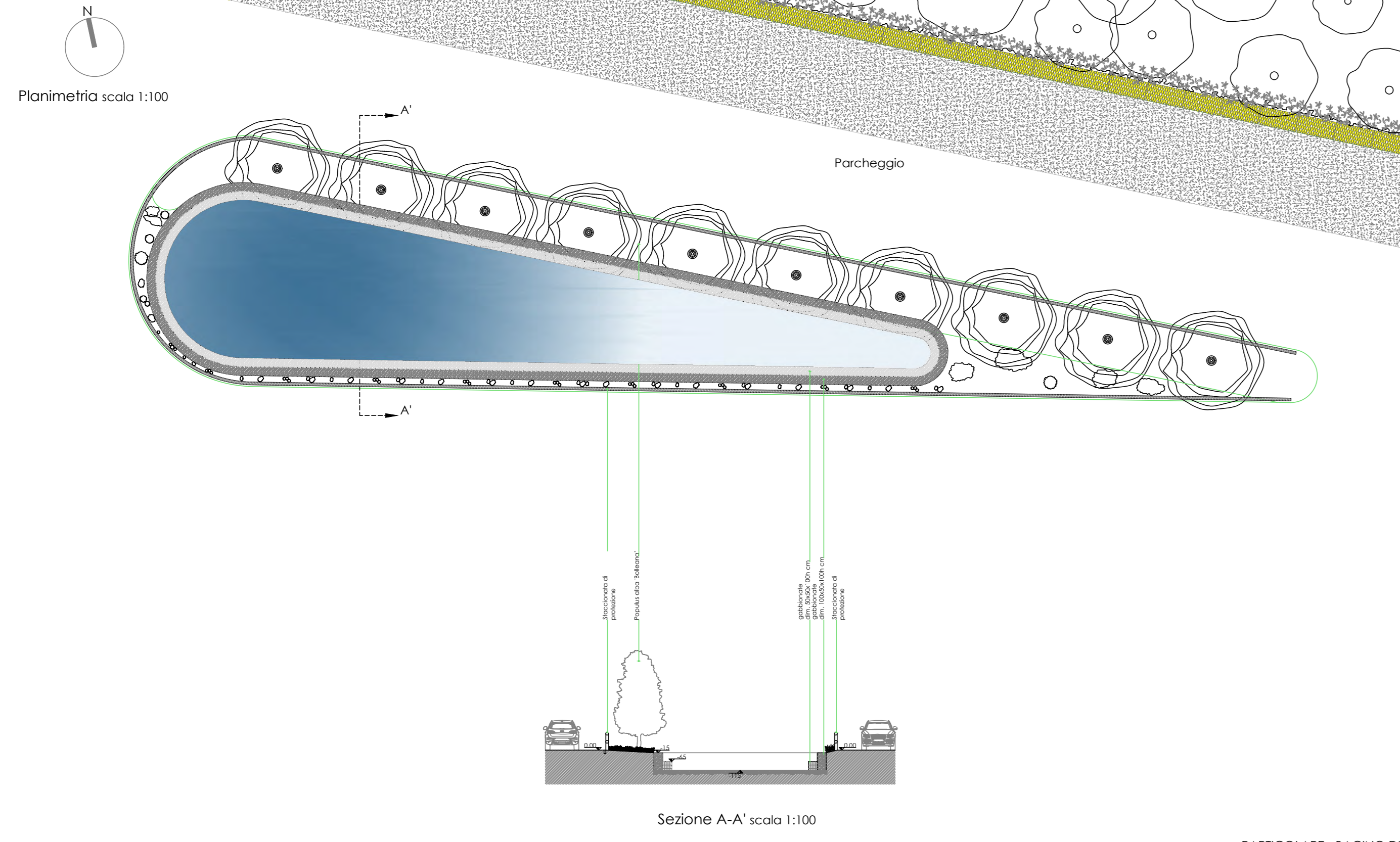
PARTICOLARE - BACINO DI INFILTRAZIONE OVEST
