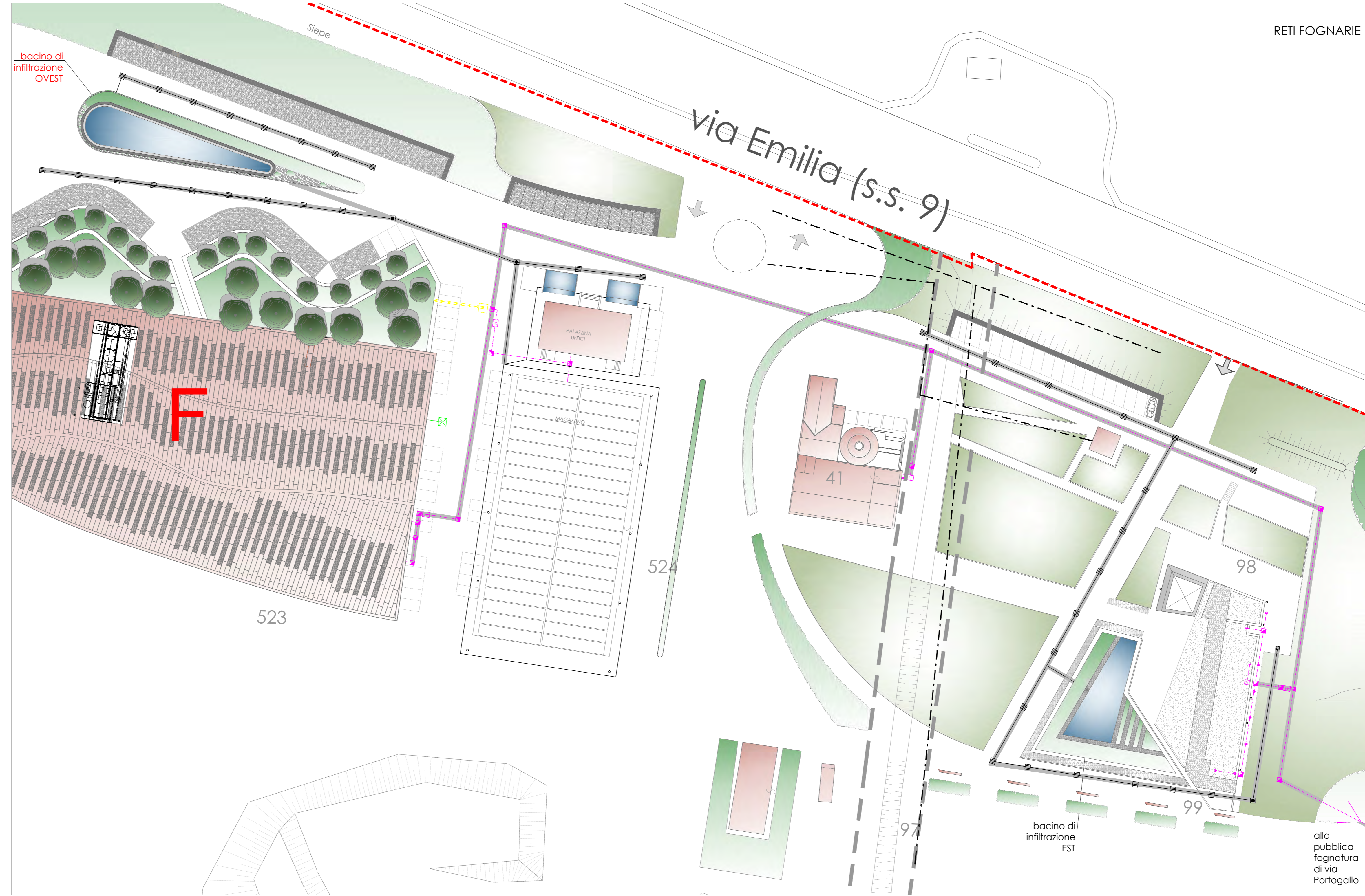
PARTICOLARE - BACINO DI INFILTRAZIONE OVEST
