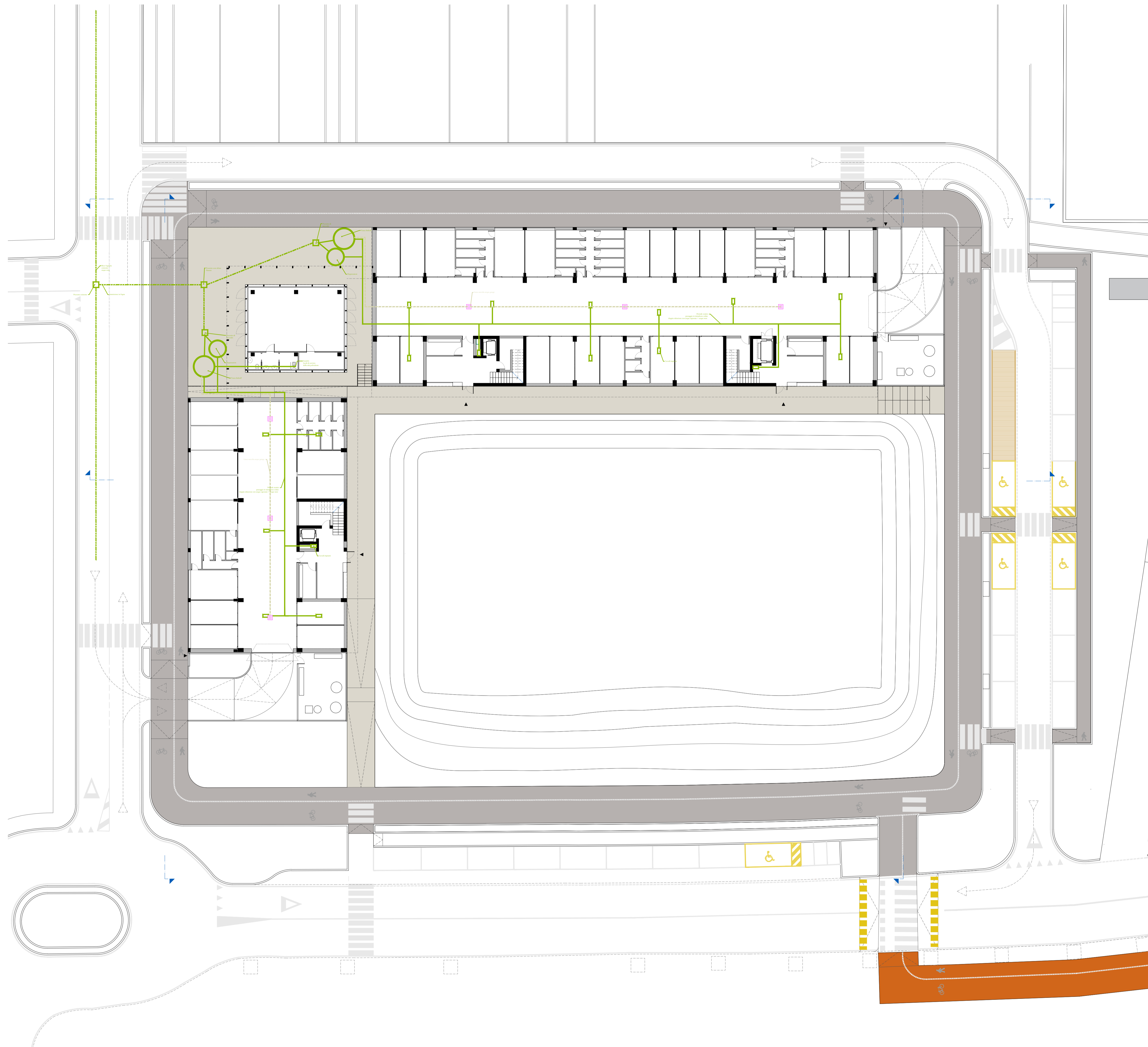
Schema fognatura acque nere, 1:200
