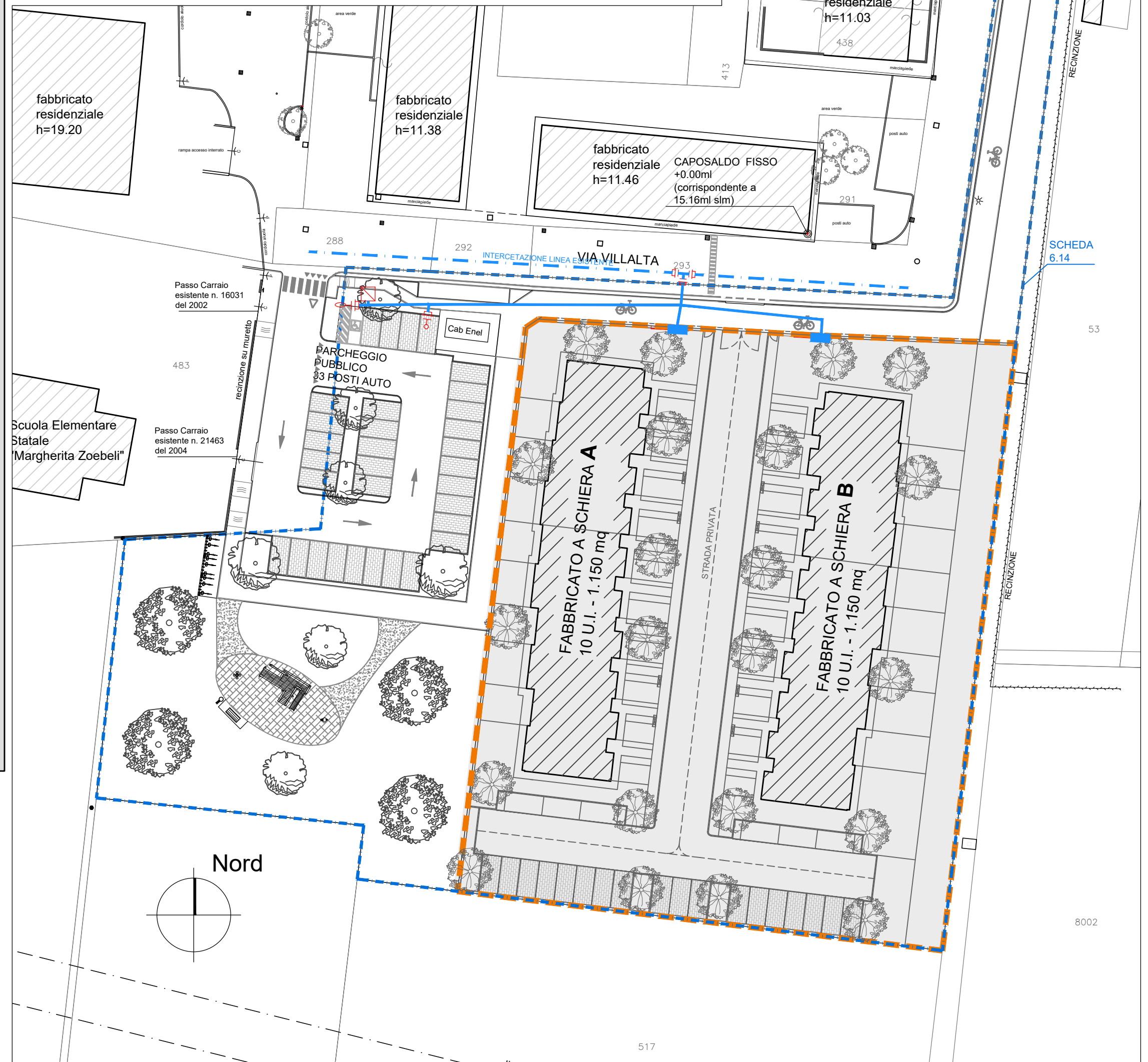
PLANIMETRIA DI PROGETTO SCALA 1:500
