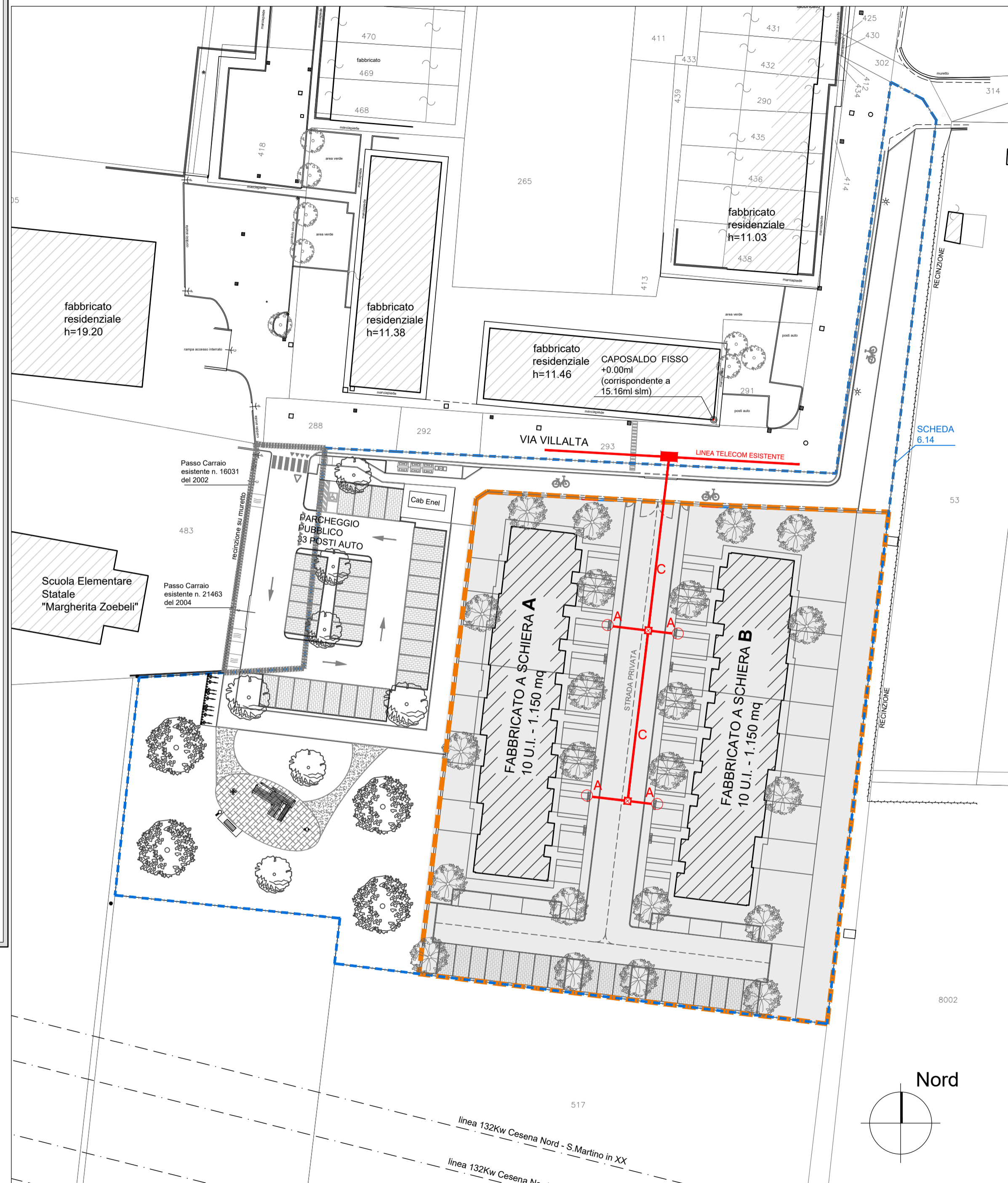
PLANIMETRIA DI PROGETTO SCALA 1:500
