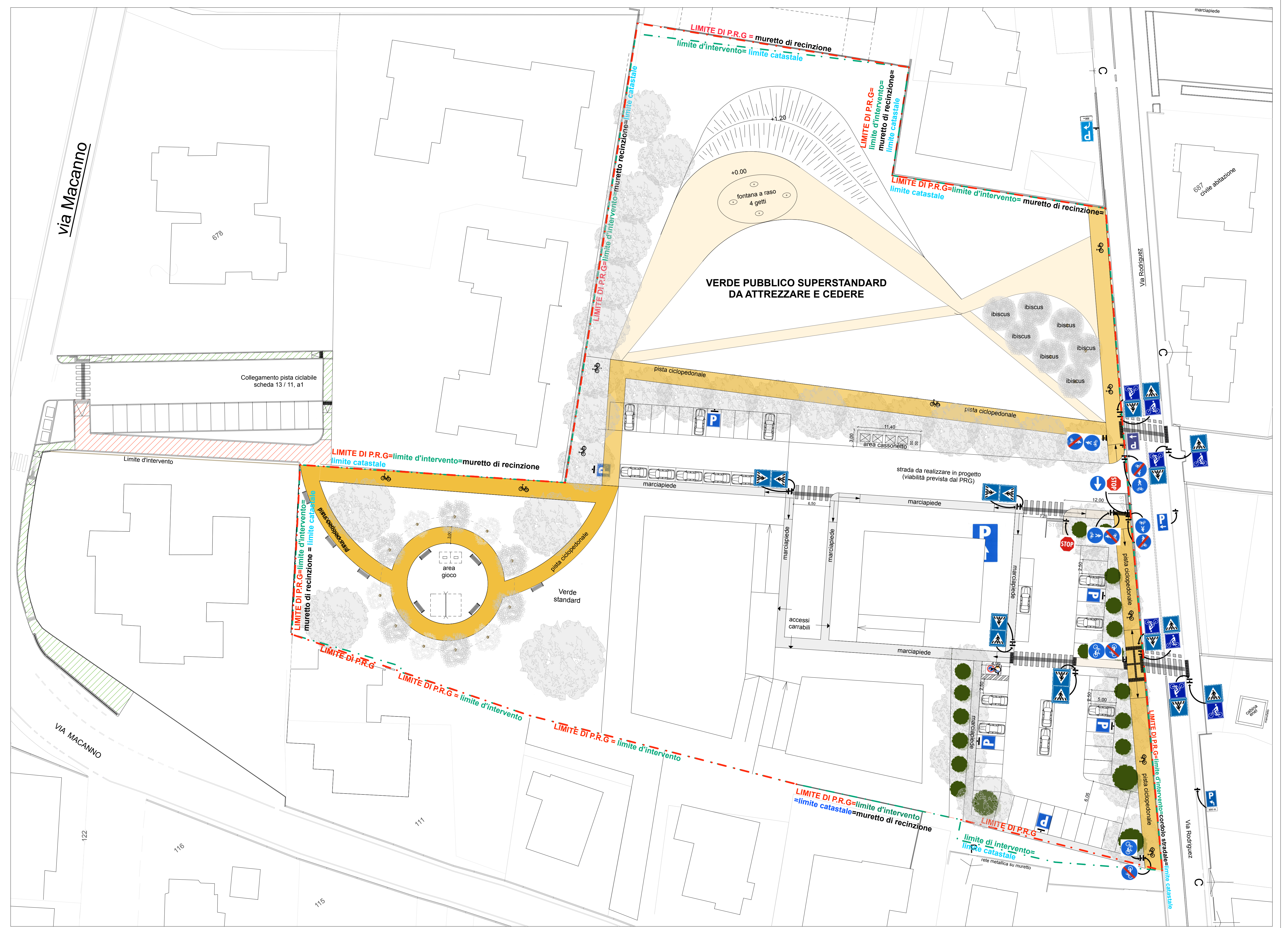
PLANIMETRIA GENERALE Scala 1:300
