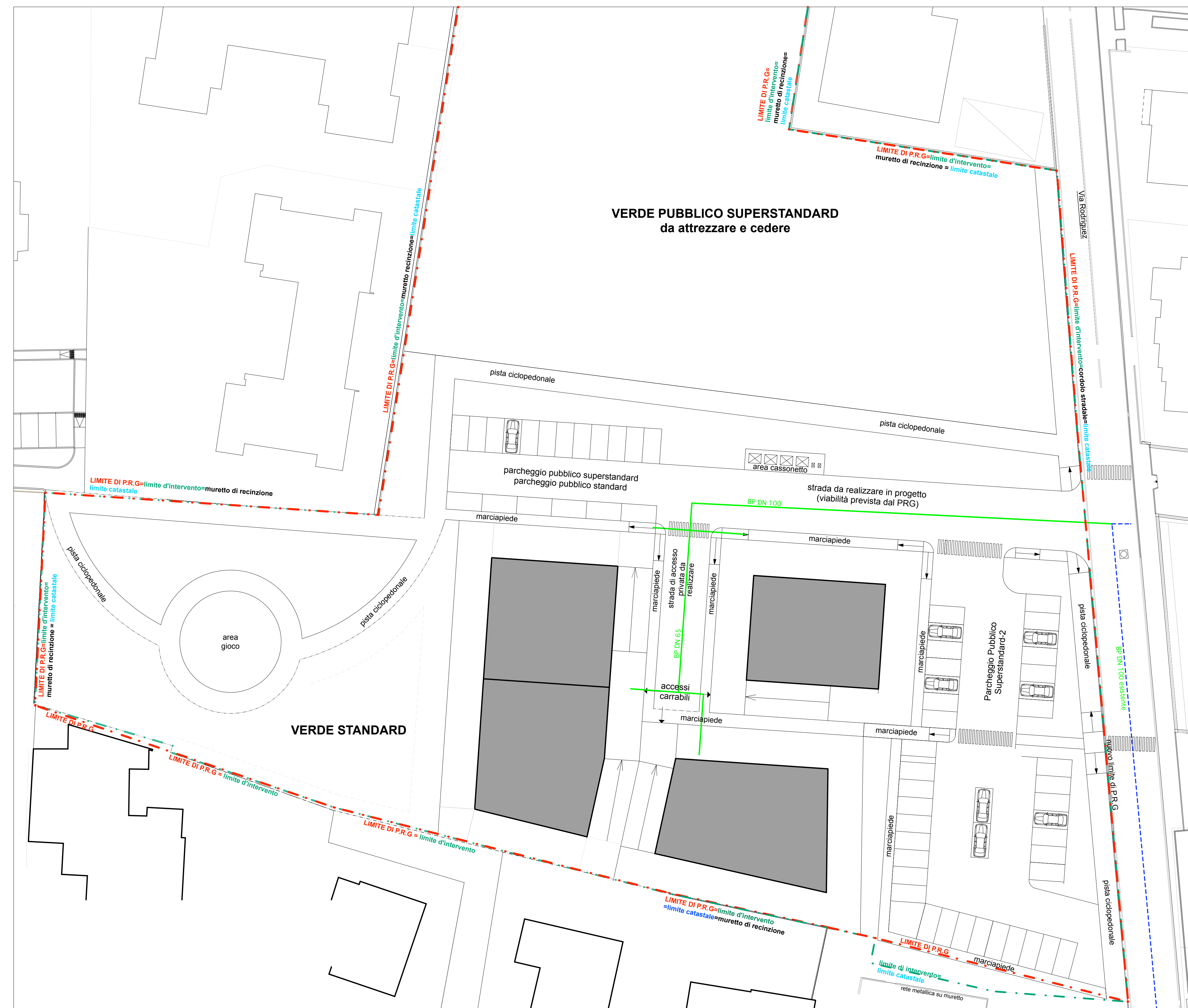
PARTICOLARE RETE GAS scala 1:20
