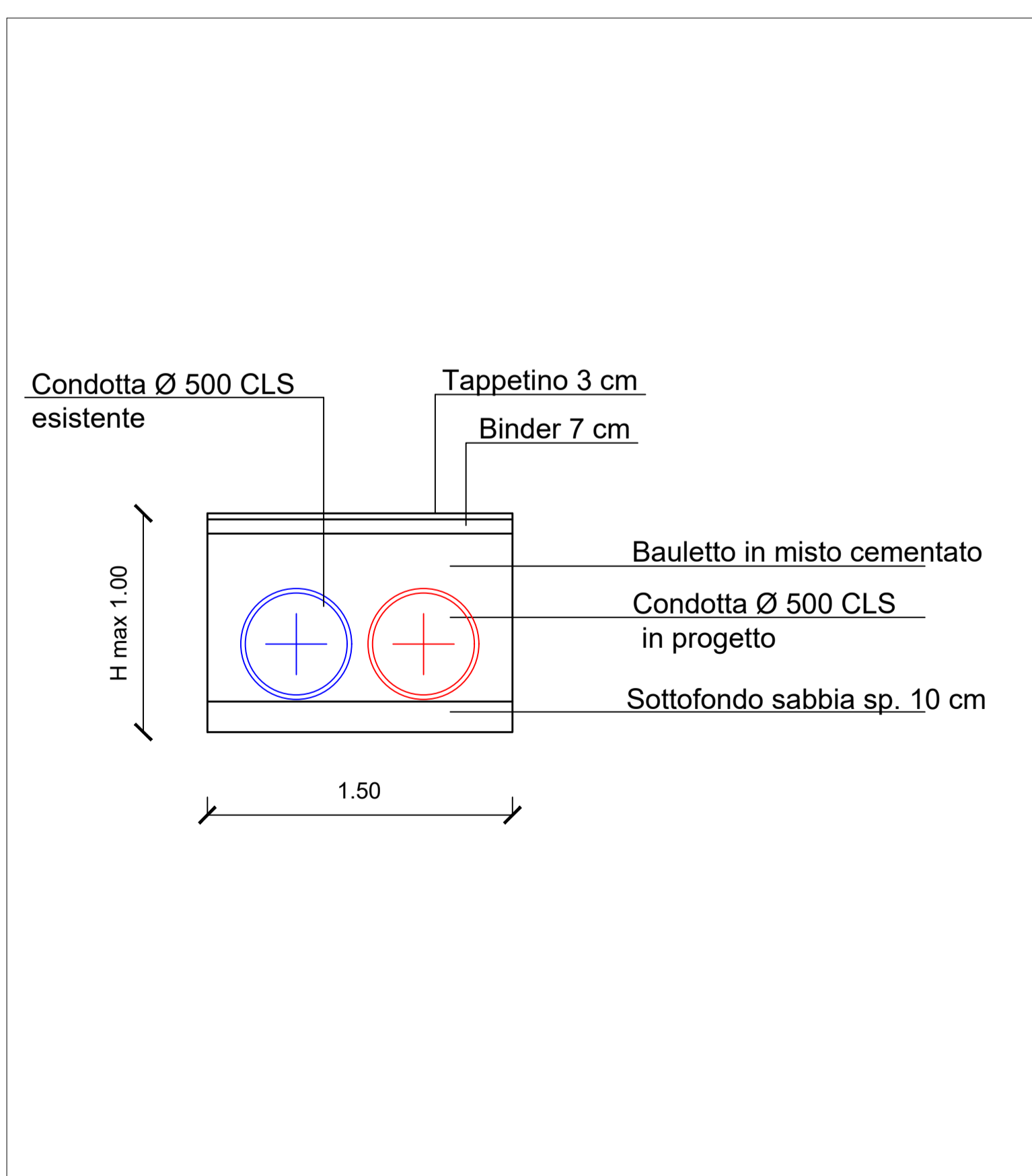
Sezione di posa tipo - scala 1:25
