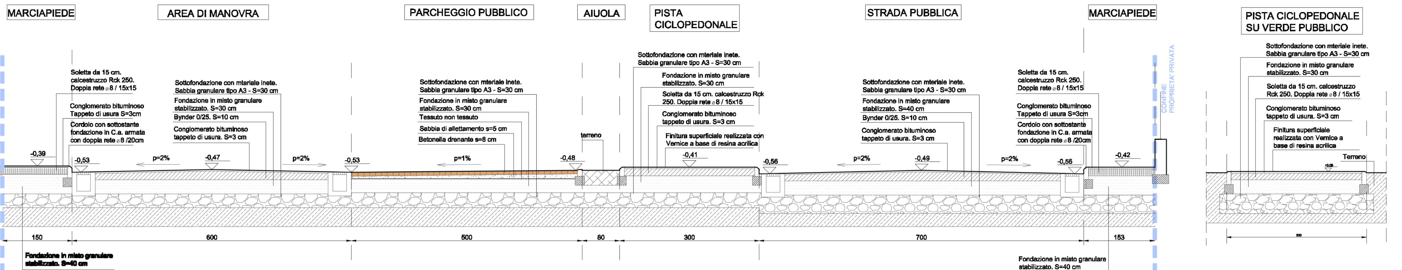
SEZIONE DI PROGETTO - AA - SCALA 1:50
