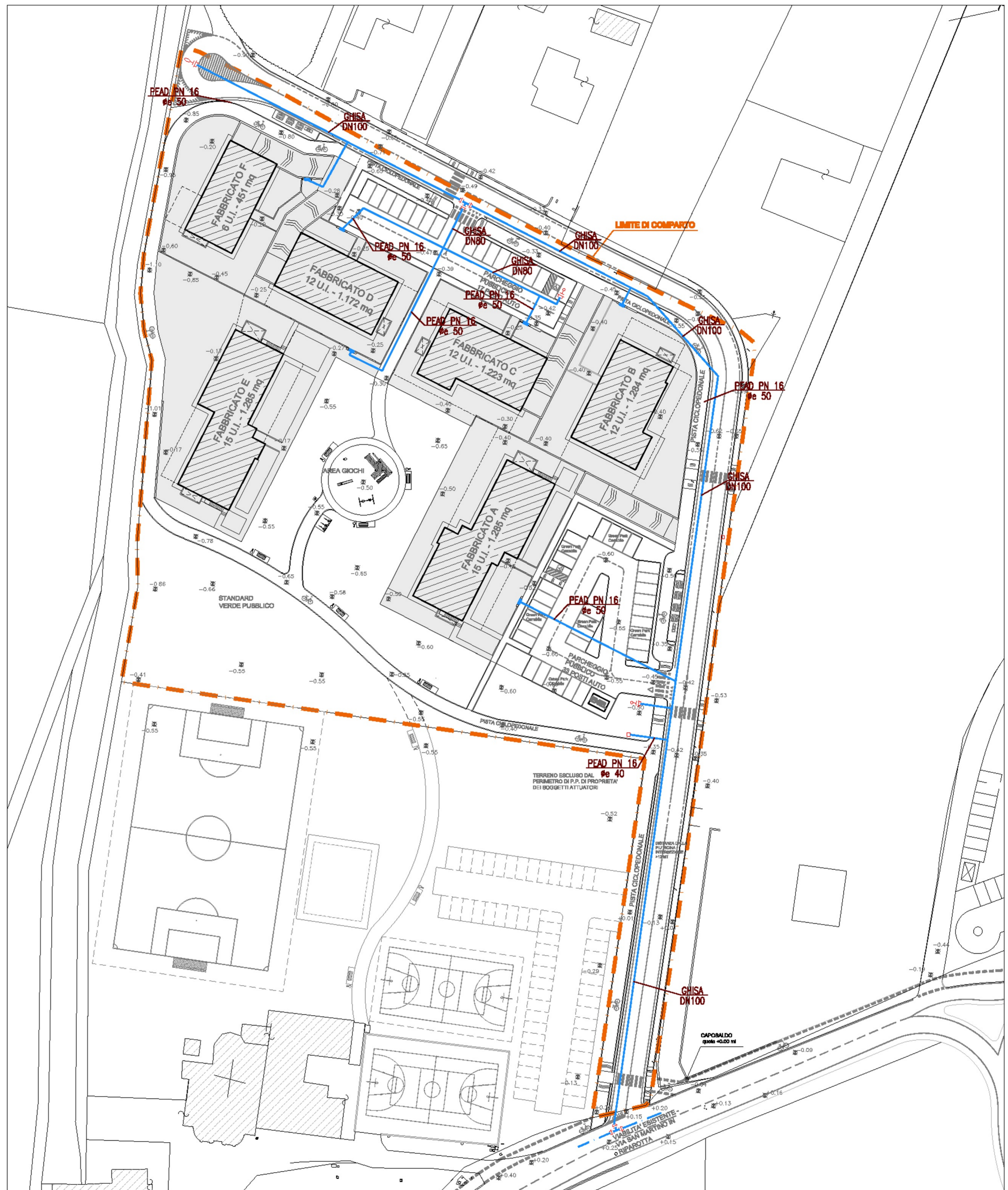
PLANIMETRIA GENERALE - SCALA 1:500
